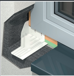
GUTMANN Entwässerungsmodul DELTA
